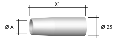
ABIMIG® A 405 LW
