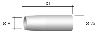
ABIMIG® A 305 / 355 LW
